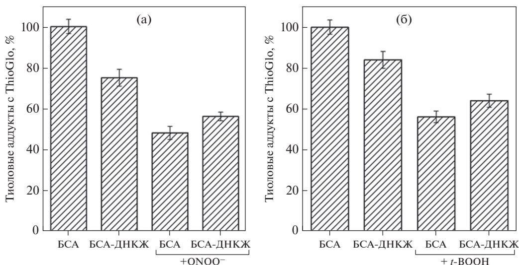
Рис. 6. Влияние образования БСА-ДНКЖ на окисление Cys34 БСА пероксинитритом (а, БСА : \text{ONOO}^- = 1 : 10) и t\text{-BOOH} (б, БСА : t\text{-BOOH} = 1 : 25).
