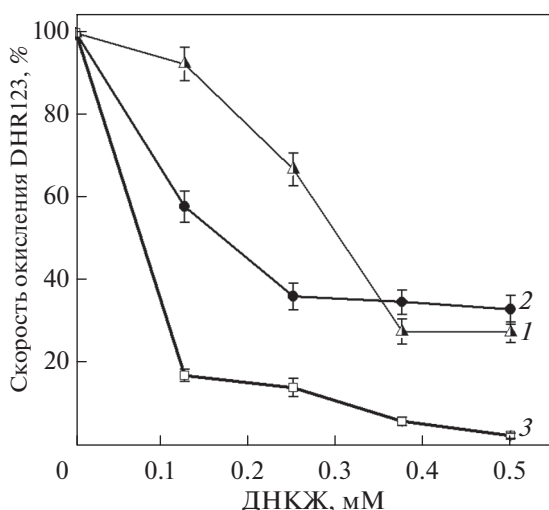
Рис. 5. Влияние низкомолекулярных ДНКЖ с тиоловыми лигандами на скорость окисления дигидрорадамина пероксинитритом, образующимся при декомпозиции SIN-1: 1 — AcCys-ДНКЖ, 2 — GS-ДНКЖ, 3 — LA-ДНКЖ. Скорость окисления дигидрорадамина в контрольном варианте (без добавок ДНКЖ) принимали за 100%.
